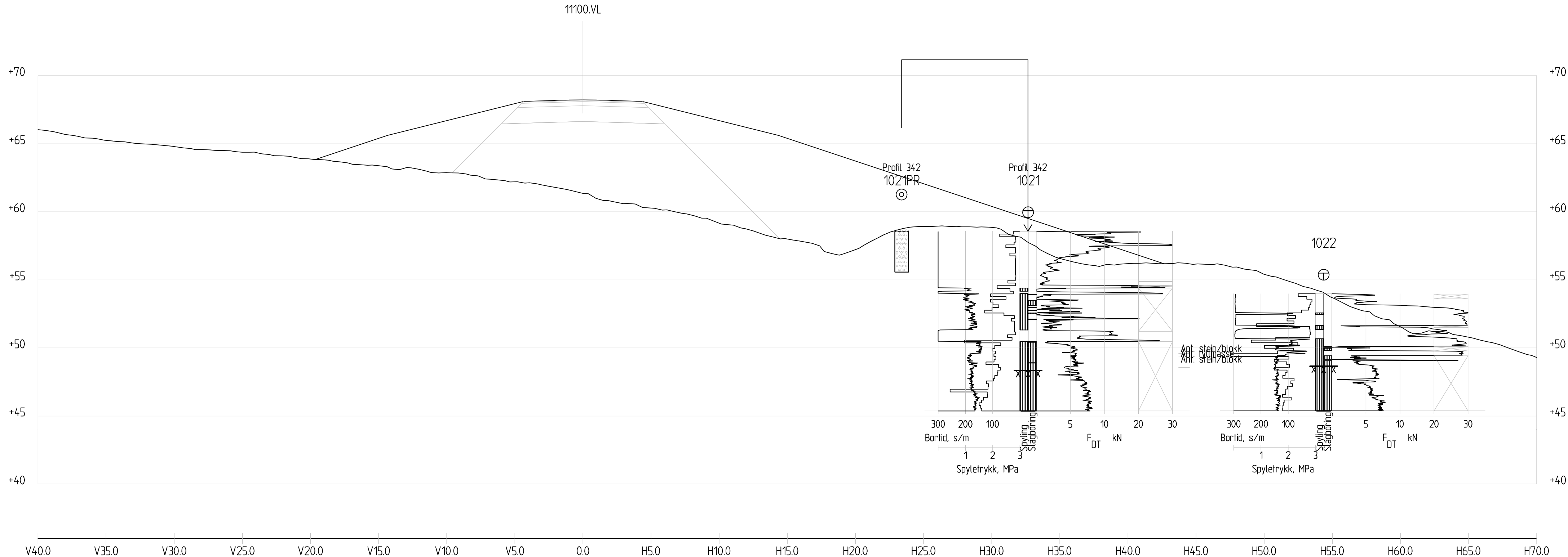
Profil 350 1 : 200
