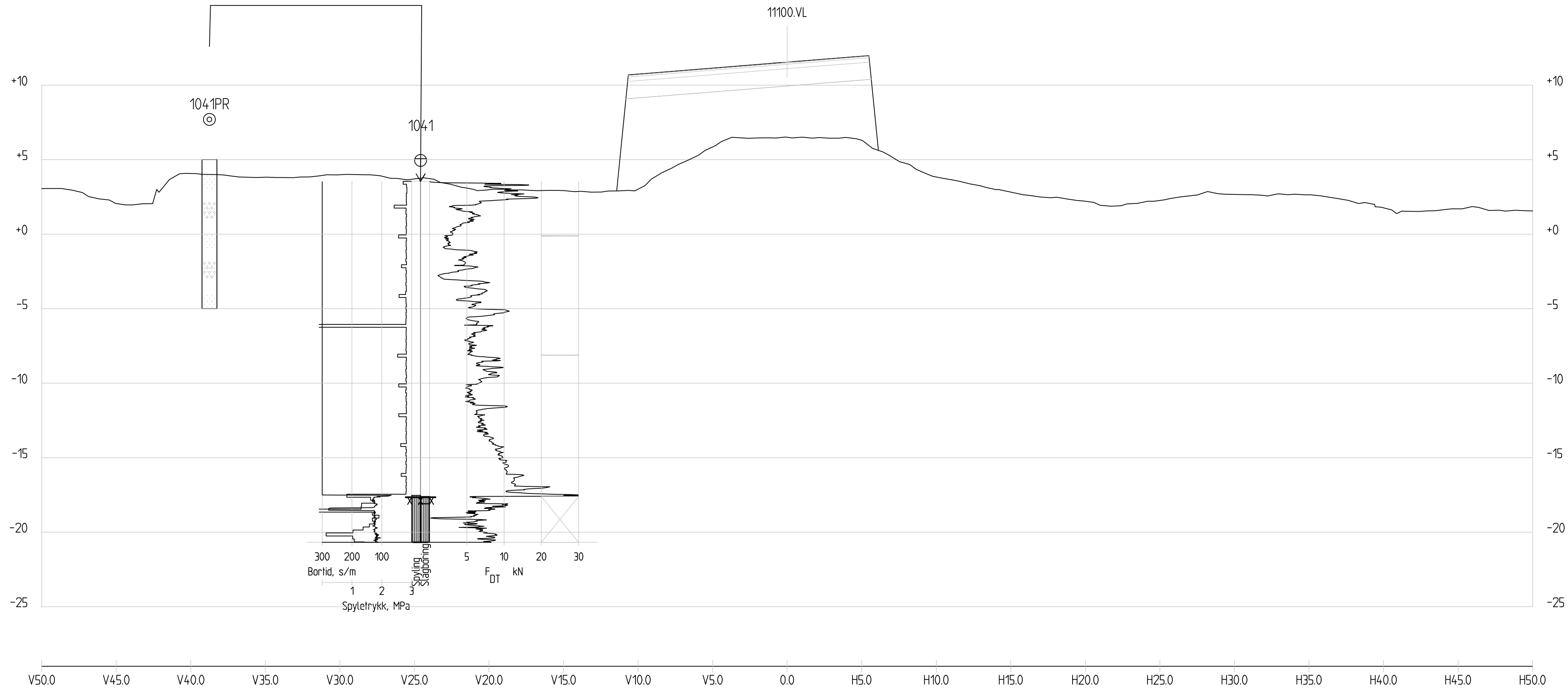
Profil 2370 1 : 200
