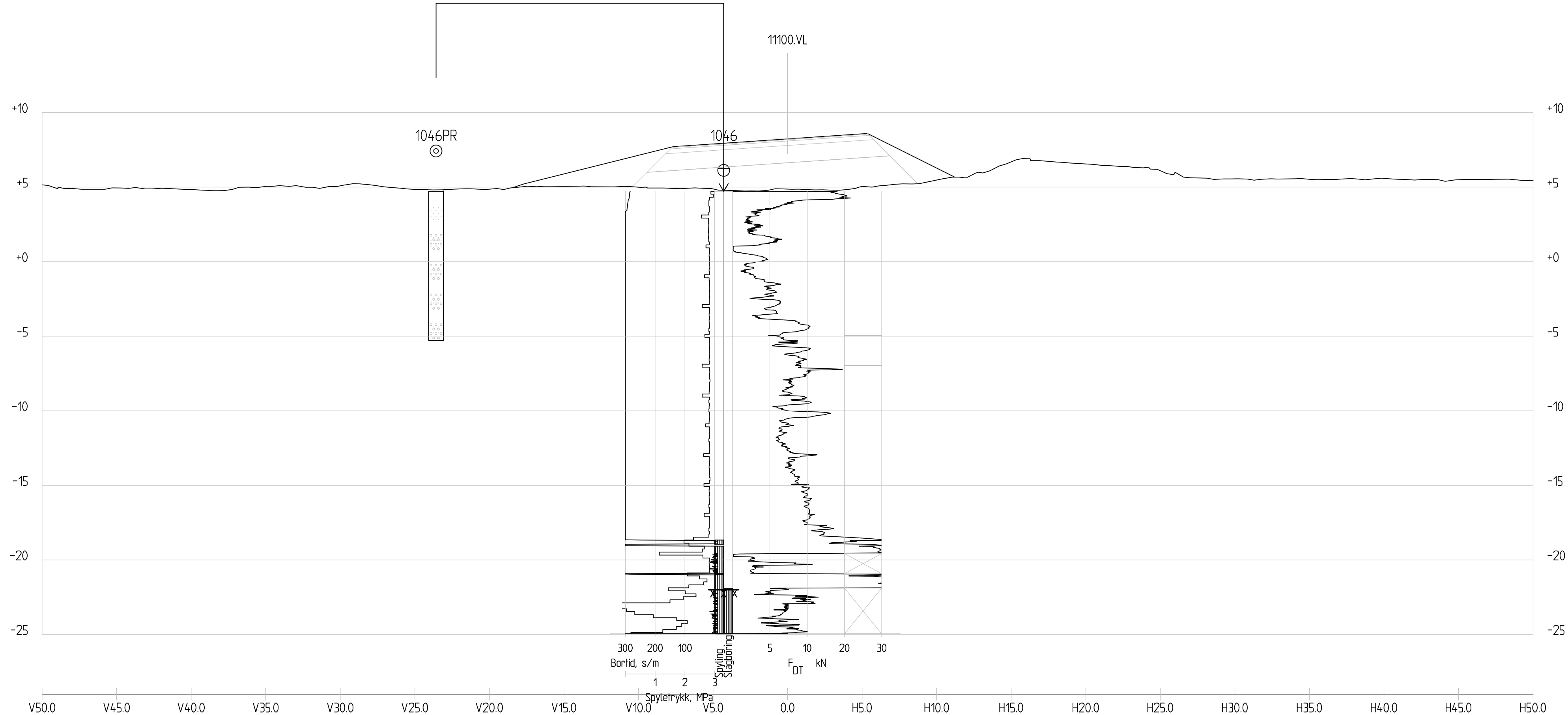
Profil 2670 1 : 200
