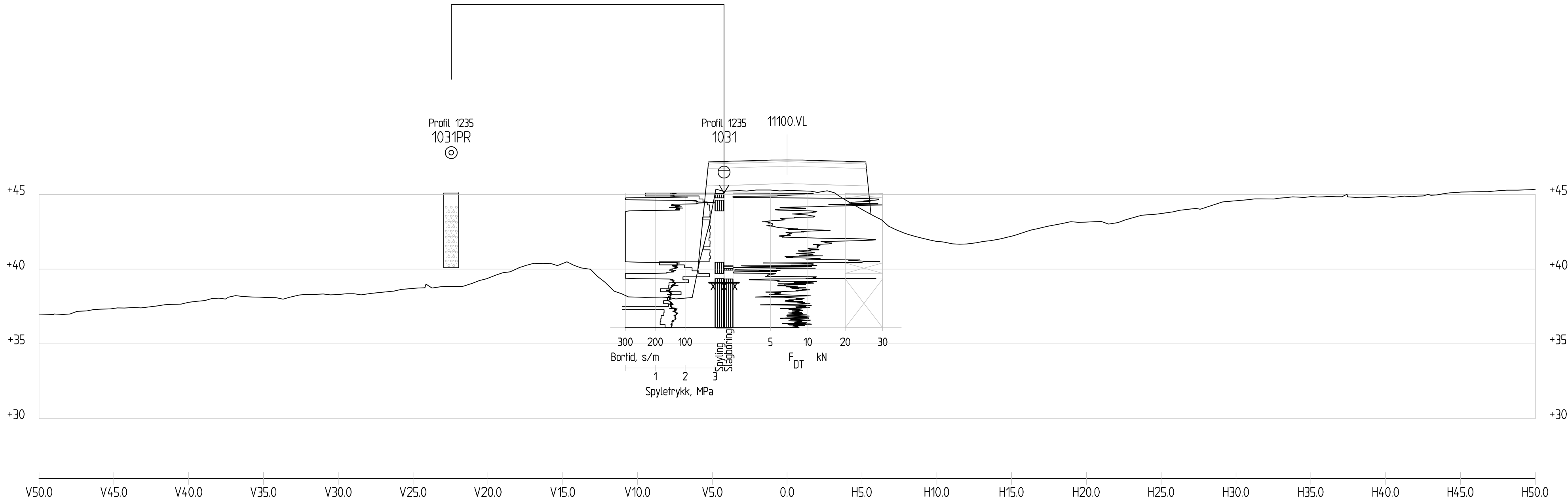
Profil 1230 1 : 200
