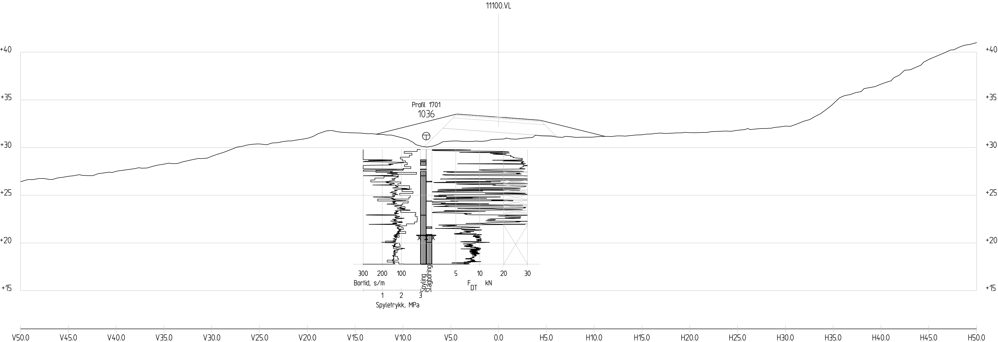
Profil 1700 1 : 200
