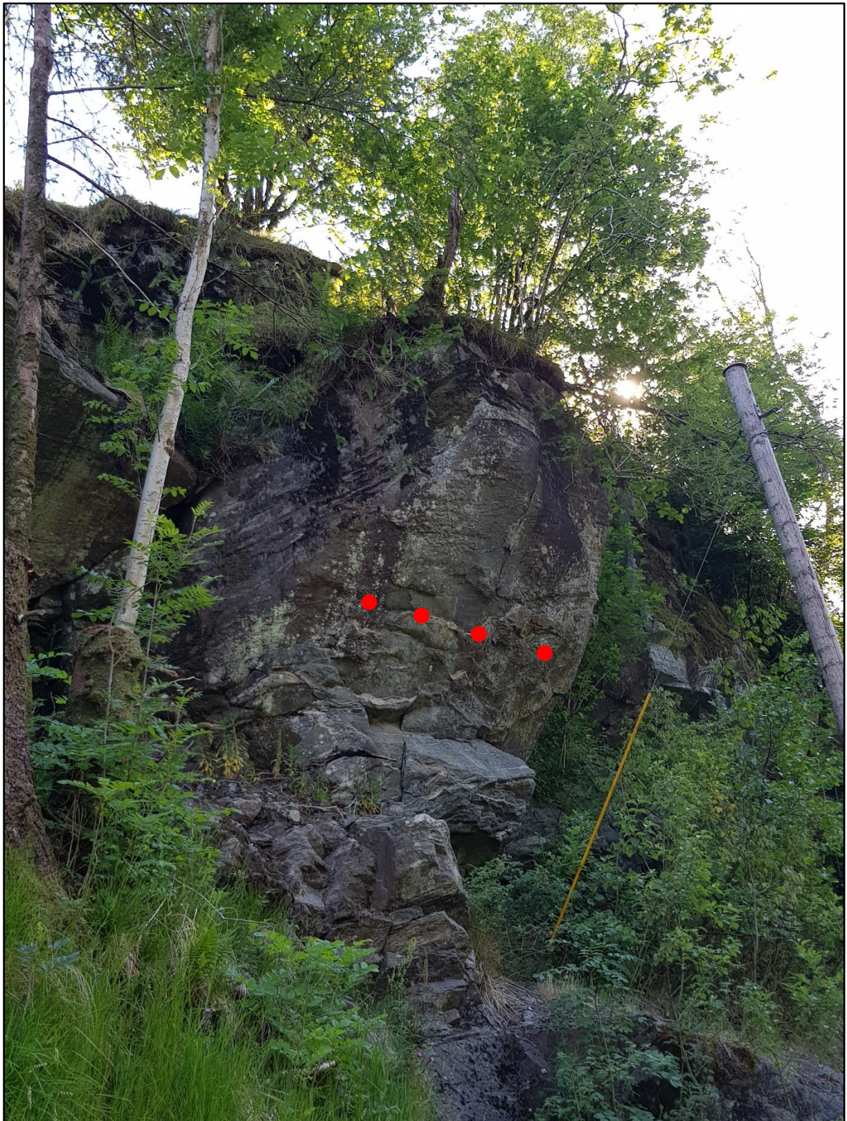
Figur 2: Stort overhengande parti i bersgråninga. Det anbefales å sikre dette partiet med 4stk ø32mm 6m lengde, alternativt Ischebeck 40/16.
