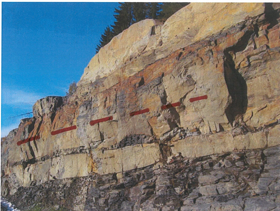
”Mage” på fjell sikres med en 3 m lang bolt pr 4 m langs vegen
